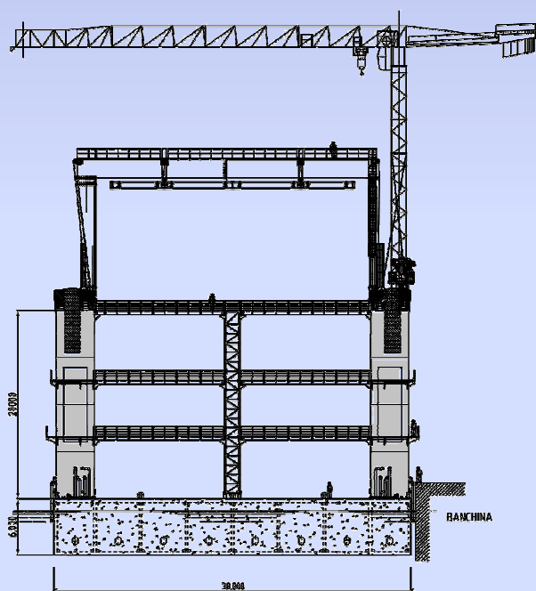
VISTA TRASVERSALE
