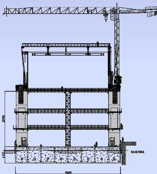
VISTA TRASVERSALE
